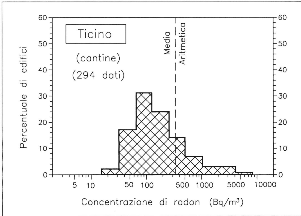
Fig. 8 Distribuzione statistica dei valori della concentrazione di radon negli scantinati in Ticino (294 dati la cui media aritmetica è 328 Bq/m 3 ). Dati aggiornati al 1989 (Bosco Gurin escluso).
