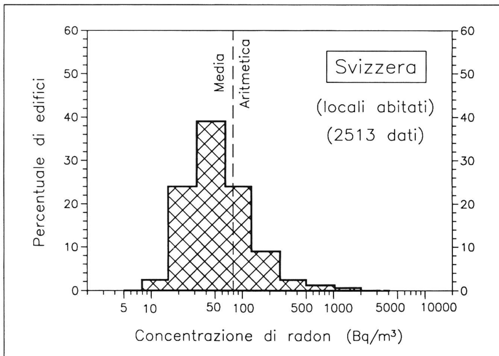
Fig. 9 Distribuzione statistica dei valori della concentrazione di radon nei locali abitati in Svizzera (2513 dati la cui media aritmetica è 81 Bq/m 3 ). In 3 % degli edifici la concentrazione supera i 250 Bq/m 3 , mentre nell'1.2 % i 500 Bq/m 3 . Dati aggiornati al 1989 esclusi quelli della campagna cantonale ticinese 89/90.
