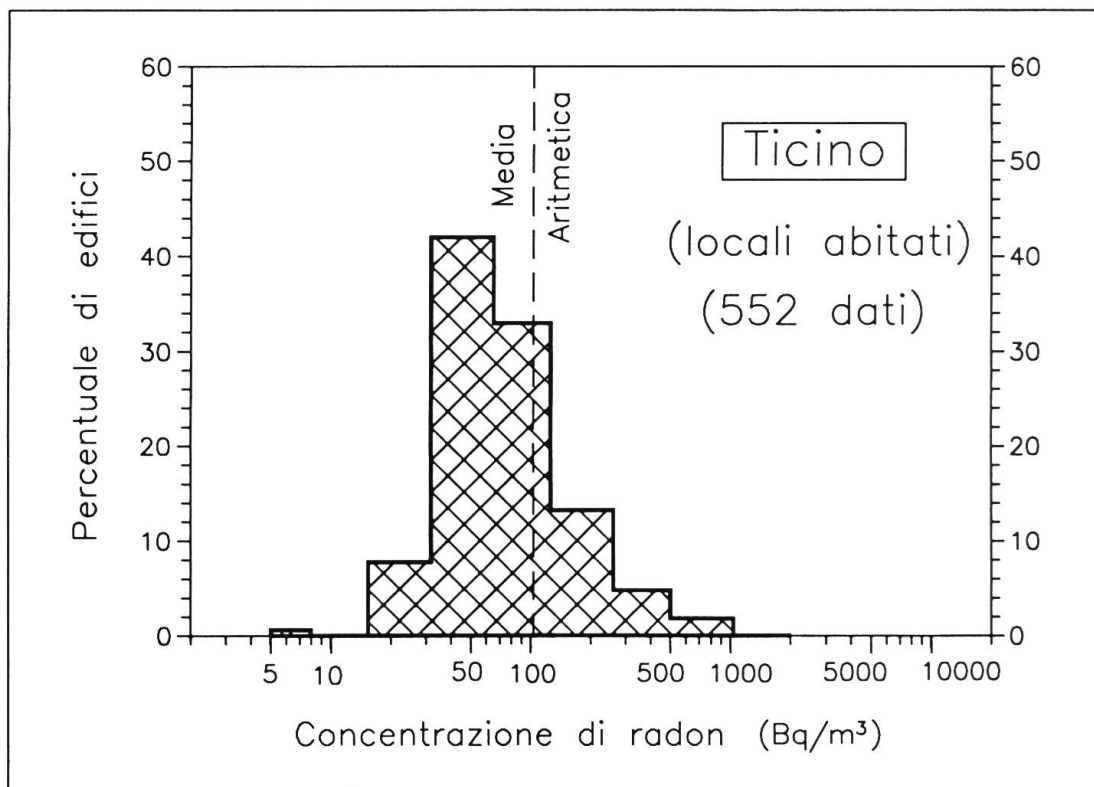
Fig. 7 Distribuzione statistica dei valori della concentrazione di radon nei locali abitati in Ticino (552 dati la cui media aritmetica è 101 Bq/m 3 ). In 6 % degli edifici la concentrazione supera i 250 Bq/m 3 , mentre nell'1.7 % i 500 Bq/m 3 . Dati aggiornati al 1990 (Bosco Gurin escluso).
