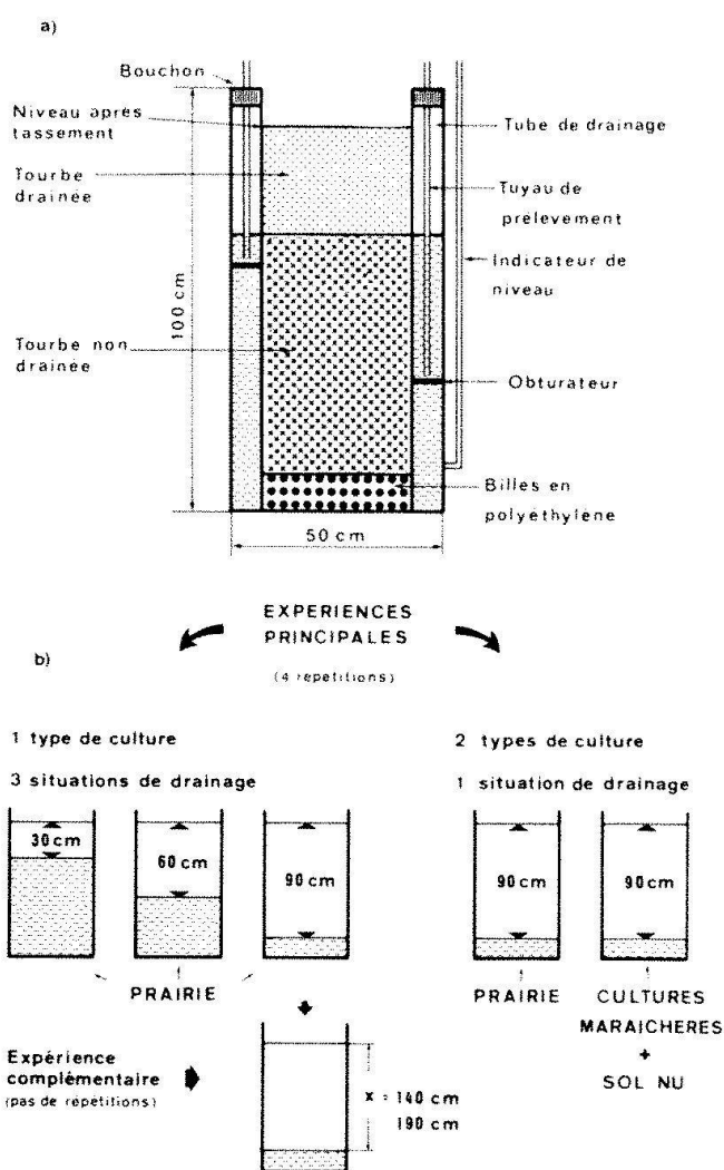
Figure 1. Dispositif expérimental.
