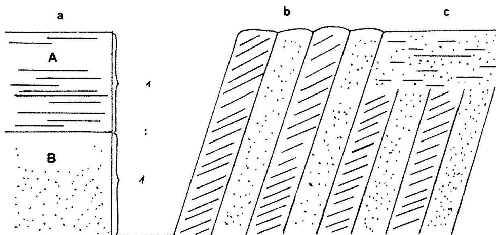
Abb. 1: Schematische Wirkungweise des Tiefpflügens. A. Moorboden, B. Sand/Lehm Unterboden, a: vor dem Tiefpflügen, b: nach dem Tiefpflügen, c: Inkulturnahme der gemischten Ackerkrume.
