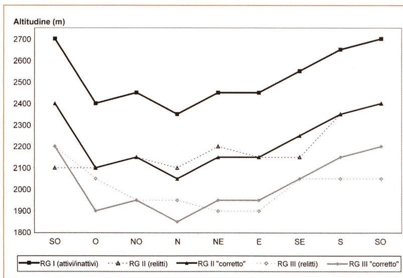
Figura 2.37 – Limite inferiore del permafrost discontinuo per ogni generazione di rock glaciers.
