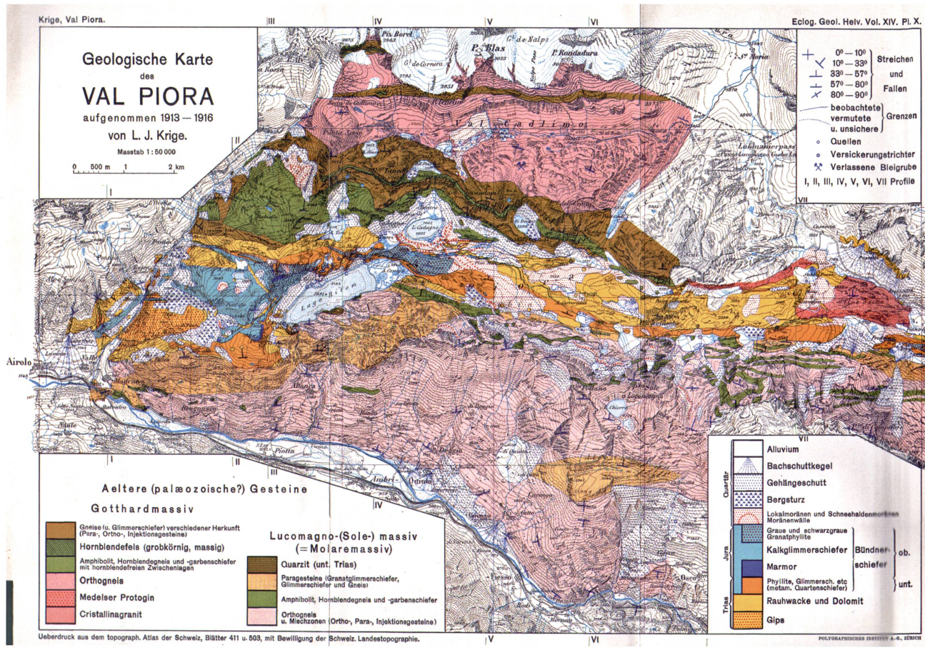
Fig. 4 - La carta geologica a scala 1:50'000 di Leo Krige (1918) copre una vasta area dell'Alto Ticino, dalla Val Canarà ad Acquacalda. Nelle grandi linee la carta è valida a tutt'oggi e torna la base di carte e testi geologici pubblicati in seguito (Presnšek et al. 1934, Nicoli et al. 1936, Antonini in questo volume).
