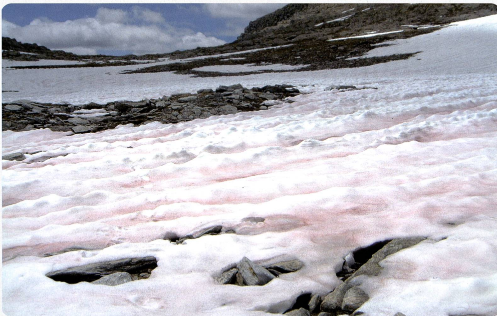
Fig. 1 – "Neve rossa" in località Piatto della Miniera tra la Val Piora e la Val Cadlimo a circa 2540 m s.l.m. (foto M. Tonolla)
