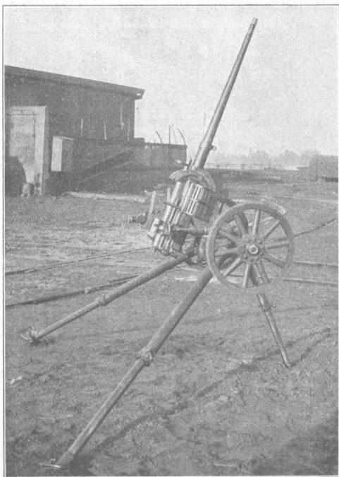
Abb. 7. Tank- und Fliegerabwehr-MG. (holl. Industrie en Handelsmaatschappij 20 mm). 7. Mitr. pour la défense contre tank et contre avion.
