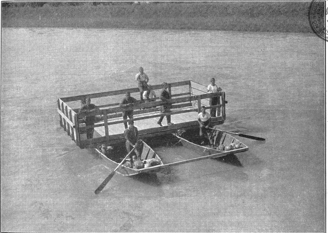
Talfahrt eines leichten Fährgliedes bei Verlegung der Uebergangsstelle. Descente d'une petite portière-volante en changeant le lieu de traversée.
