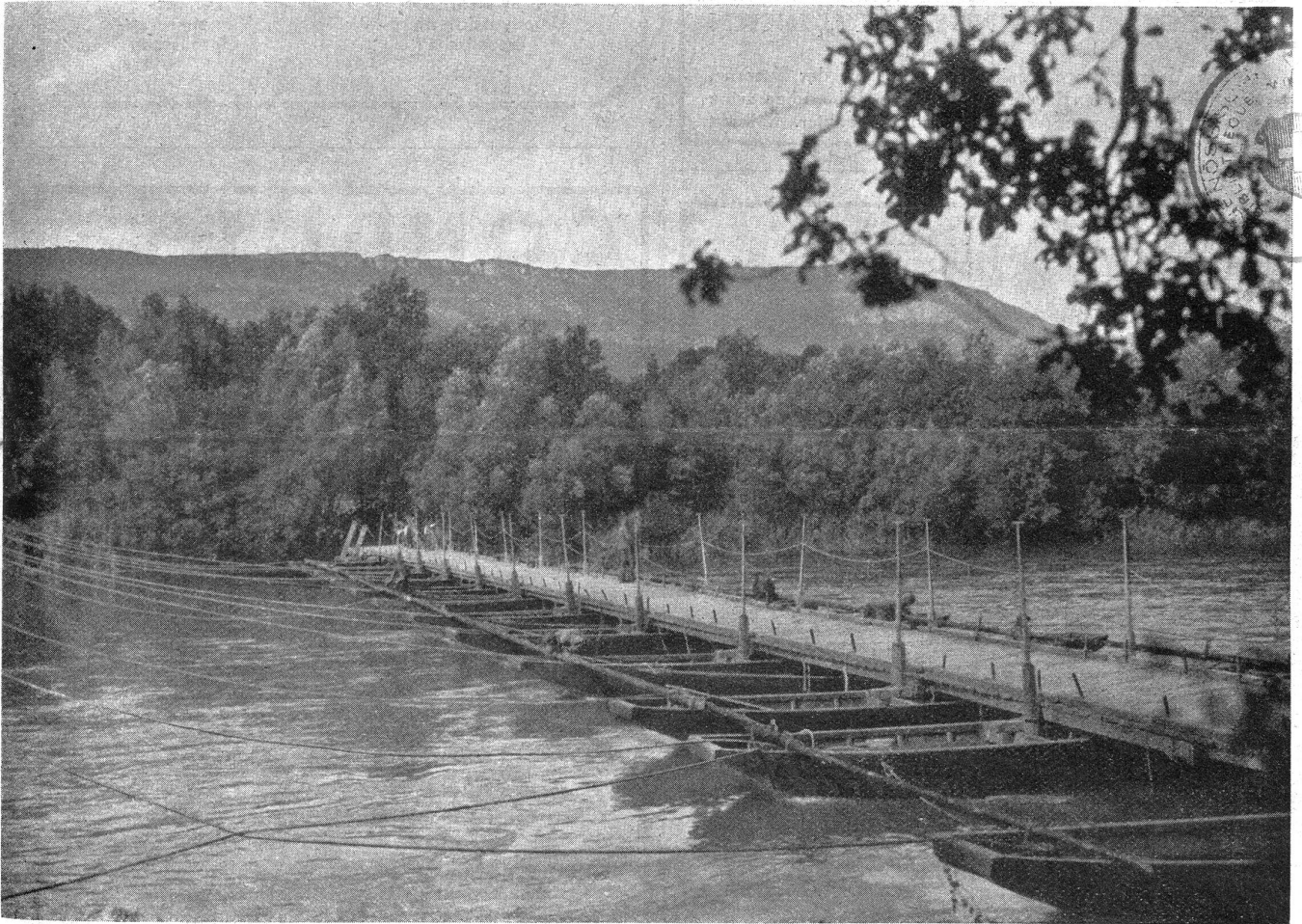
Schertaubrücke. — Die Pontons hängen an einem über den Fluss gespannten Drahtseil, dem sogen. Schertau. Pont à cinquenelle. — Les pontons sont accrochés à un câble dit cinquenelle tendu sur la rivière.
