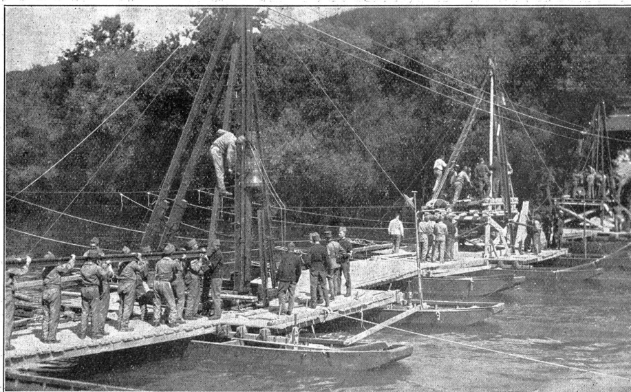
Construction d'un pont par les pon- tonniers; Travaux de bantages
