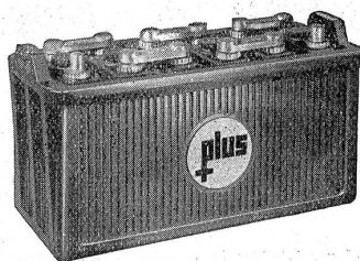
Autobatterie Type 6 E 5, 12 Volt, 75/100 Ah
