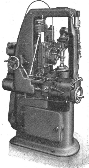
Halbautomatische Universal-Abwälz- Räderfräsmaschine Nr. 2
