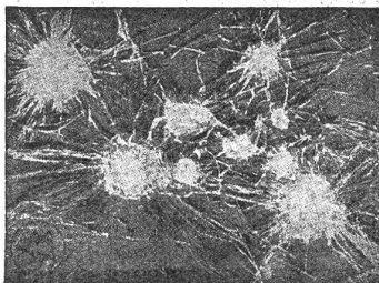
Zerschossenes Panzerglas, 4 schichtig, 20 mm dick
