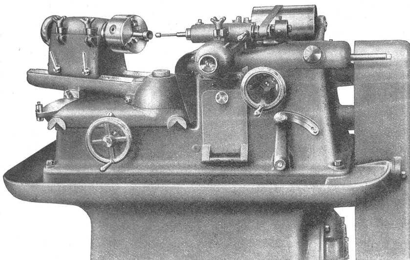
Innenschleifmaschine
