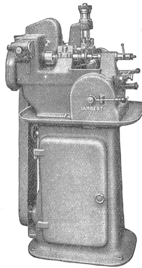
Halbautomatische Abwälzräderfräsmaschine Nr. 1 Type 75
