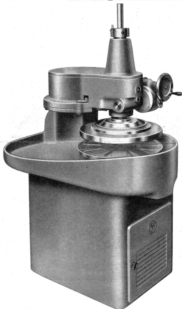
Hochpräzisions-Läppmaschine SV 560
