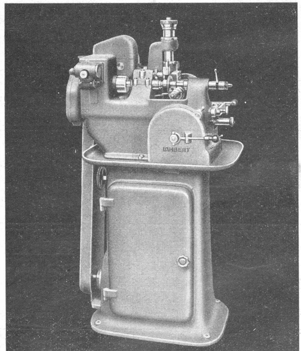
Abwälzräderfräsmaschine Type 75
