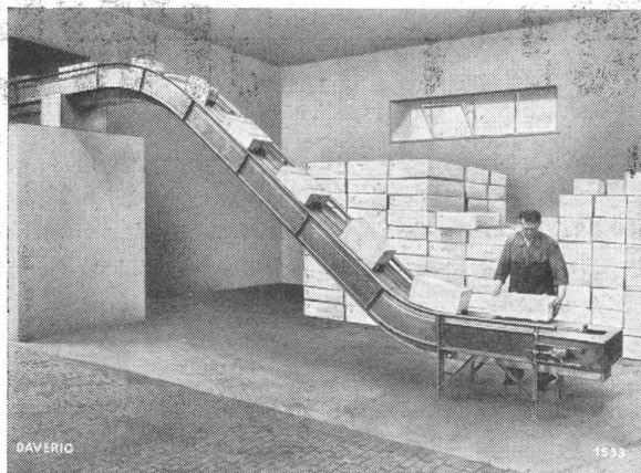
Kistentransporteur
