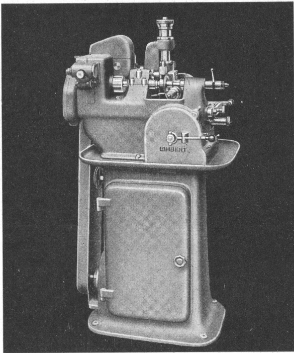
Abwärlzrüderfräsmaschine Type 75 MASCHINEN FÜR UHRENFABRIKATION UND APPARATEBAU S. LAMBERT A.G. GRENCHEN-SCHWEIZ
