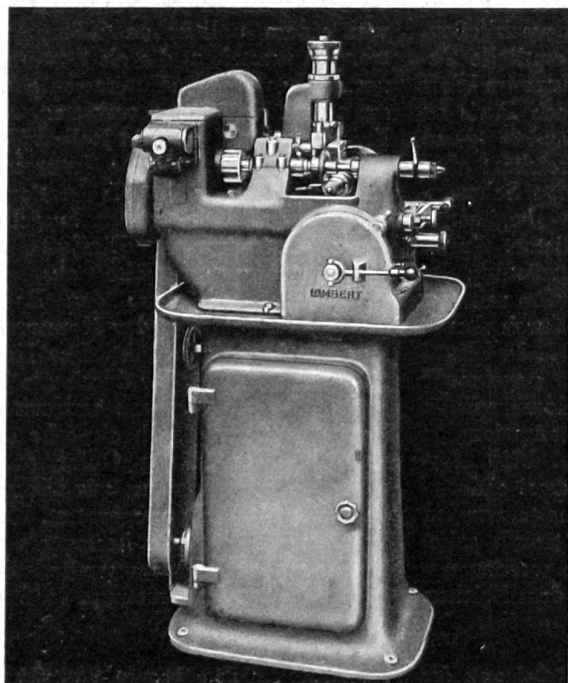
Abwälzräderfräsmaschine Type 75
