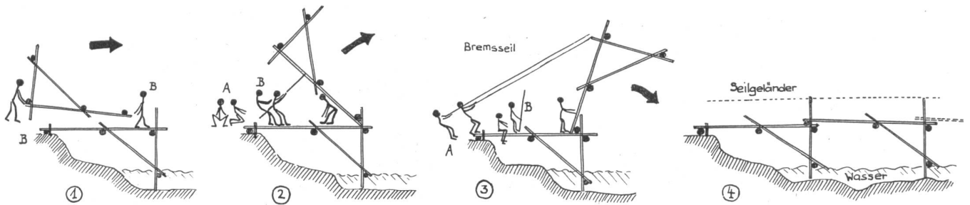
Einbau des Klappsteges
