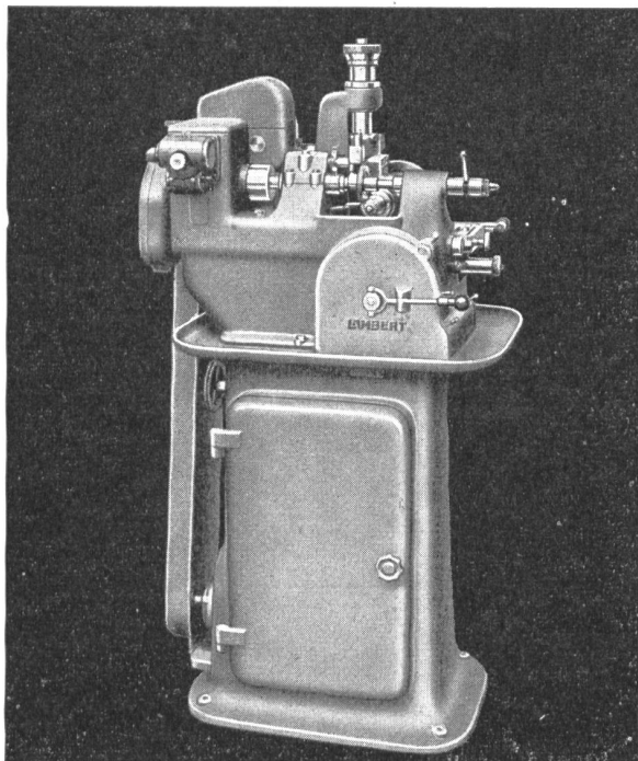
Abwälzräderfräsmaschine Type 75
