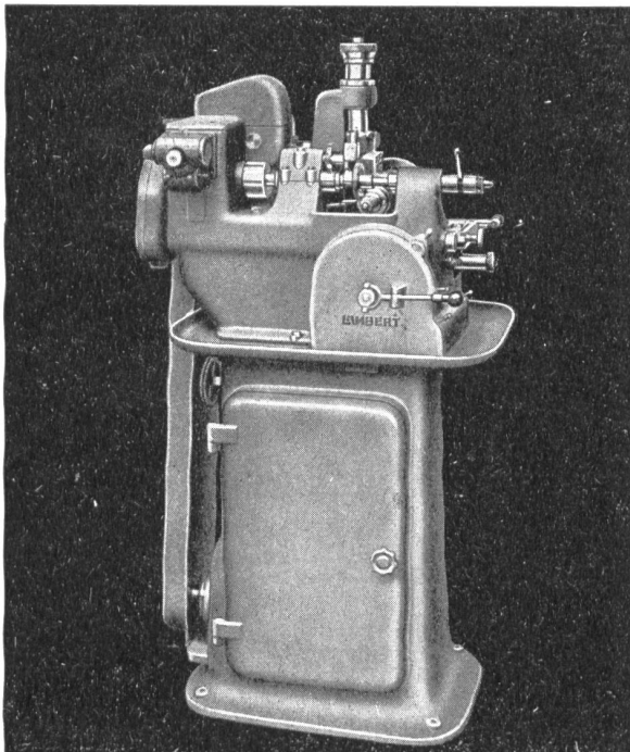
Abwälzräderfräsmaschine Type 75
