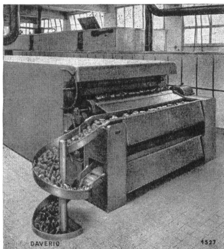
Transportanlage für Brot
