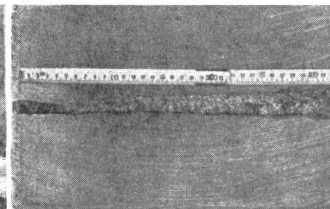
Wirkung der Hohlladung 8-cm-Panzerrakete
