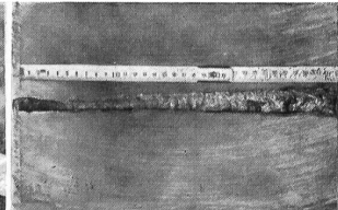
Wirkung der Hohlladung 8-cm-Panzerrakete
