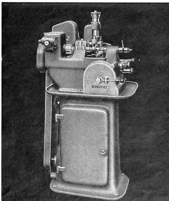
Abwälzräderfräsmaschine Type 75
