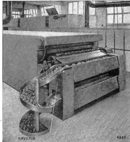
Transportanlage für Brot
