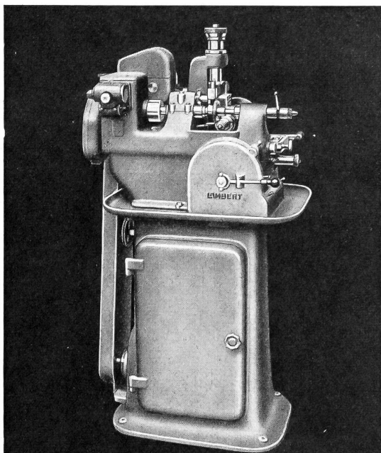
Abwälzraderfräsmaschine Type 75
