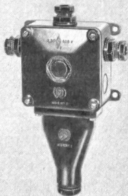
Bakeltdose mit angebautem, druckfestem Endverschluss
