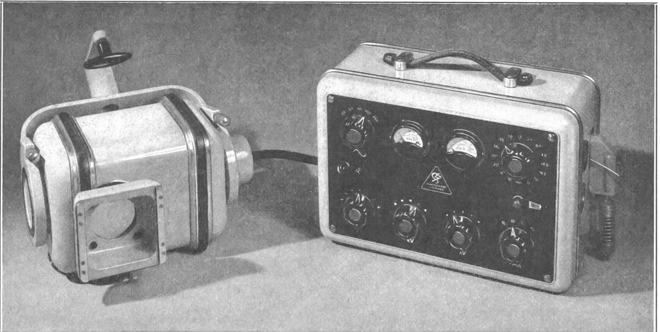
«MONOBLOC»-Eintank-Röntgen-Apparat 40 mA, 85 kVs, einer der leistungsfähigsten Kleinröntgenapparate der Welt
