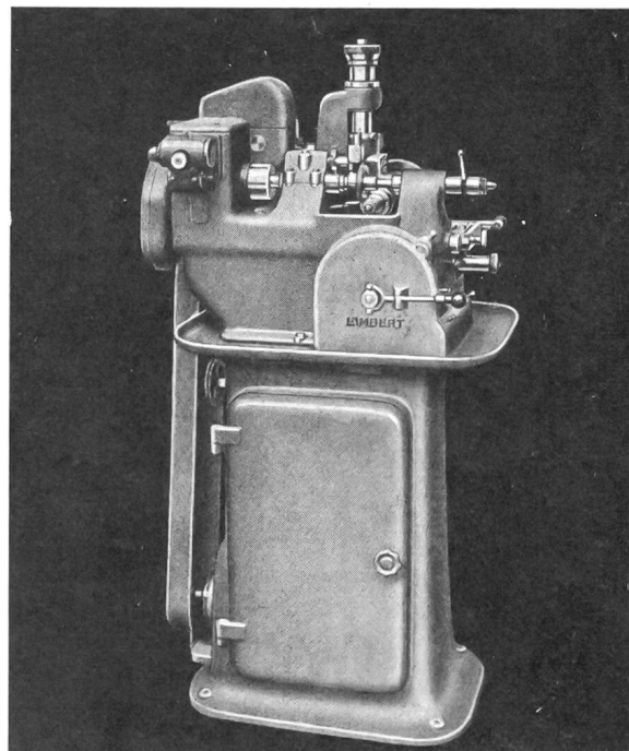
Abwälzräderfräsmaschine Type 75
