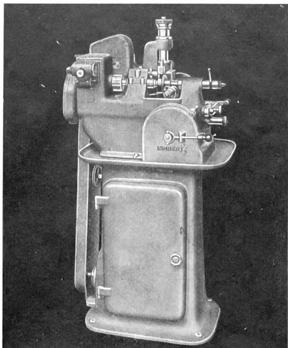
Abwälzräderfräsmaschine Type 75
