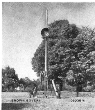
Aufbau des Antennenmastes
