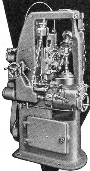
HALBAUTOMATISCHE UNIVERSAL-ABWÄLZ- RÄDERFRÄSMASCHINE
