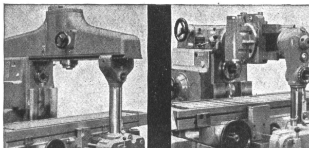
Oberarm «hvv» mit eingebauter Vertikalfrässpindel
