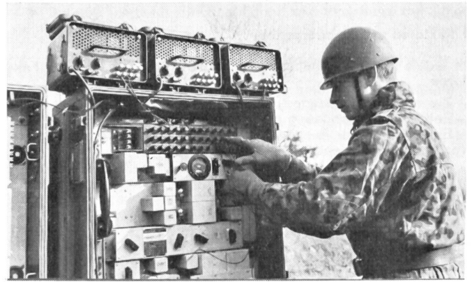
Trägerfrequenzgerät zur Mehrfachausnutzung von Leitungen
