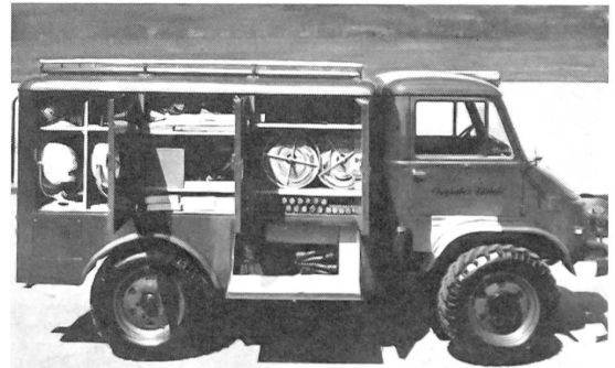
UNIMOG-S als Pionierfahrzeug
