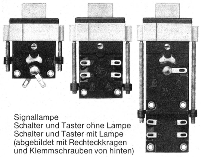
5 auswechselbare Krage- varianten zum Einbauen in runde und rechteckige Schalttafelöffnungen.
