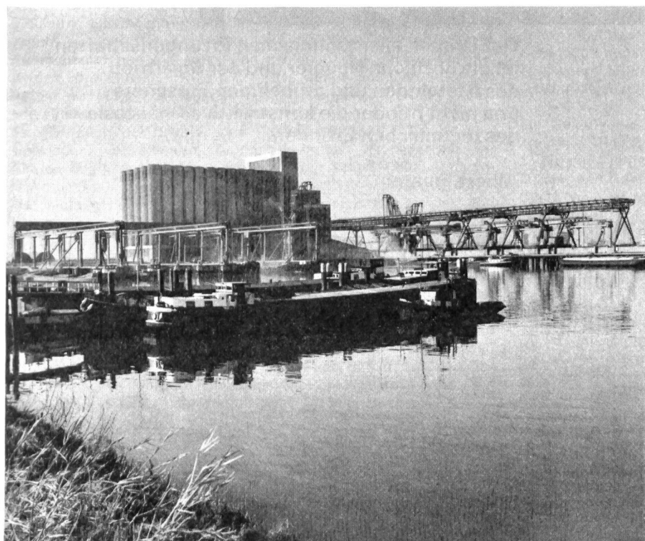
BÜHLER-Umschlags- und Siloanlage im Hafen Botlek (Rotterdam)
