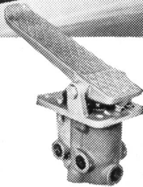
Zweikreis-Steuerventil BEKA
