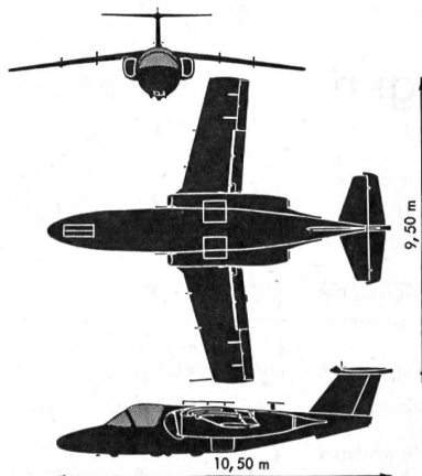
Schul- und Kampfflugzeug SAAB 105 XT
