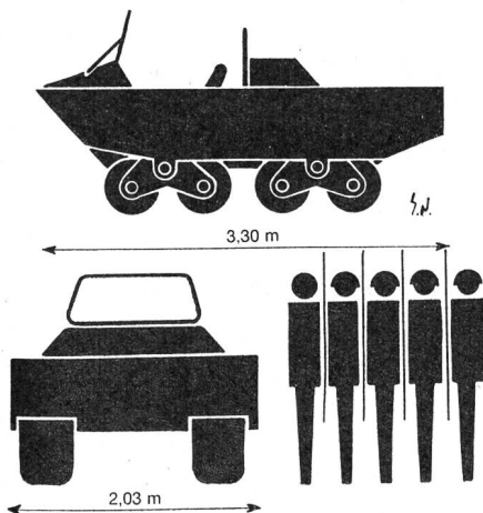
TRANSPORTFAHRZEUG LOCKHEED «TERRA STAR» (schwimmfähig)
