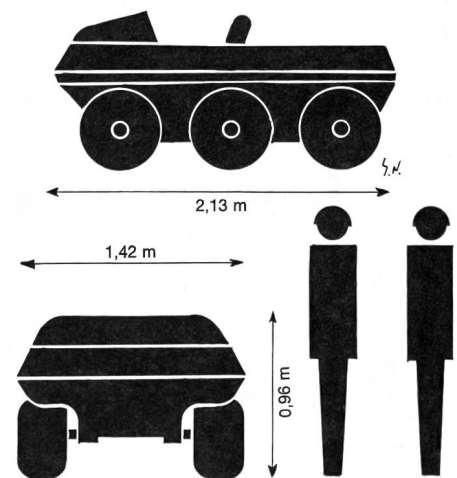
Transportfahrzeug Solo 750
