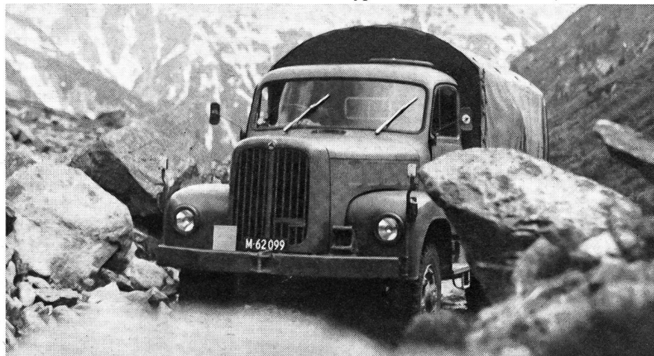
Geländegängiger Allradwagen von Saurer-Berna, Typ 2DM/2VM, seit 1964 im Einsatz als Lastwagen und Kipper.
