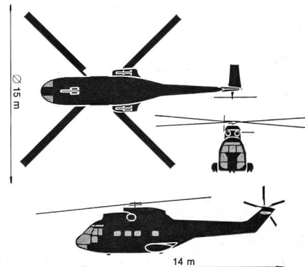
Transporthelikopter Aérospatiale SA 330 Puma
