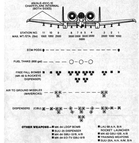
Alternative Zuladungsmöglichkeiten des Panzerjägers und Luftnahunterstützungsflugzeugs A-10
