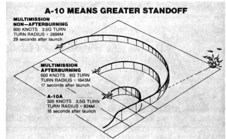
Einsatzprofil A-10 Thunderbolt II im Rahmen von Panzerabwehr-Luftnahunterstützungsmissionen (ADLG 8/79) ka
