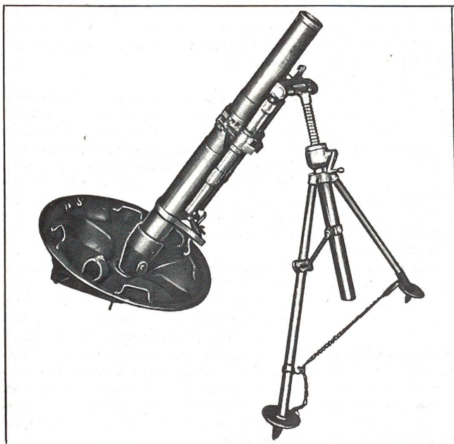
12 cm Minenwerfer. Gewicht in Feuerstellung 270 kg. Geschossengewicht 16 kg. Vo 272 m/sek. Schussweite 5,5 km. Feuergeschwindigkeit 4-6 Schuss/min. Zum Werfer gehört eine pneumatische Zweiradlafette. Zugfahrzeug: Lastwagen
