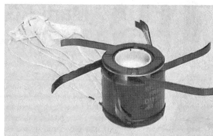
MUSPA - Splitterladung mit passiver Sensorik; über Fallschirm gebremster Flug; Bekämpfung von rollenden und startenden Flugzeugen sowie Pistenreparaturfahrzeugen.
