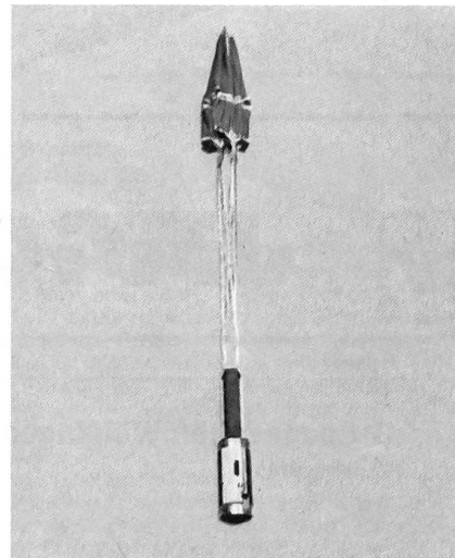
STABO - Tandemladung mit Aufschlagzünder; über Fallschirm gebremster Flug, für das Durchschlagen und Aufwerfen von Betonflächen.
