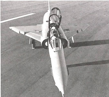
Der Stolz der South African Air Force ist zweifellos das neue Cheetah-Kampfflugzeug, das aus der Mirage III E weiterentwickelt wurde. Im Juli 1986 wurde die erste Cheetah der Öffentlichkeit vorgeführt. Hauptmerkmal sind die beiden Entenflügel über dem Luft-einlauf sowie der neugestaltete Bug mit einer in Südafrika entwickelten Avionik. In den kommenden Jahren sollen sämtliche Mirage III E/D auf den Cheetah-Standard umgerüstet werden. Diese Arbeiten werden bei ATLAS in Johannesburg durchgeführt.
