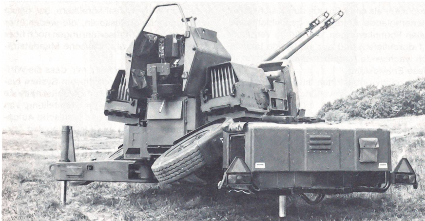
Kampfwertgesteigerte 35-mm-Fliegerabwehrkanone 63/90.
